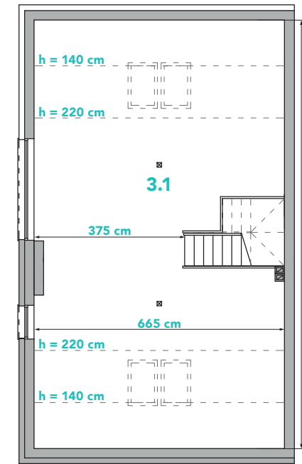
Poddasze
